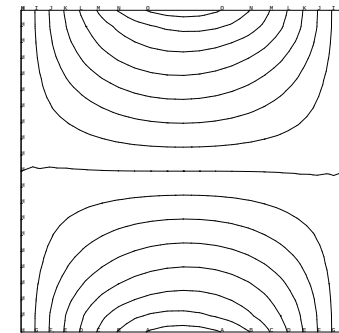
FIG. 2.4.12 – Champ de vitesse (composante u ) calculé
