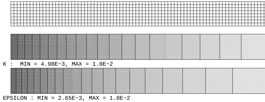
FIG. 3.1.1 – Maillage 8 \times 80 utilisé pour simuler la décroissance de la turbulence. L'entrée du domaine est constituée par le bord gauche du maillage. Isovaleurs de k et de \epsilon pour la solution convergée.
