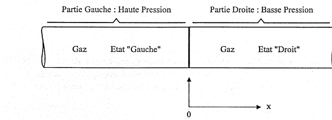
FIG. 5.1.1 – Conditions initiales du tube à choc.
