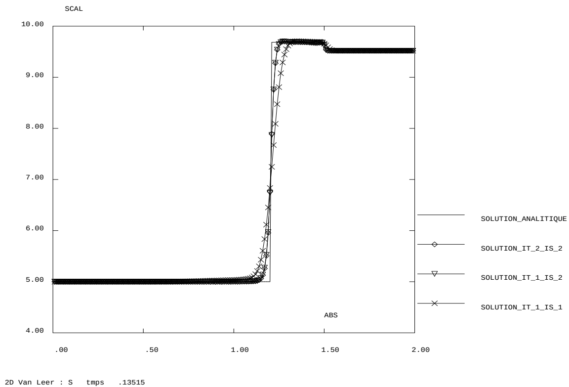
FIG. 5.1.14 – Entropie.
