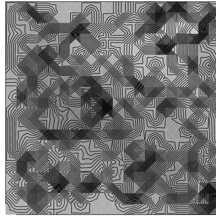
FIG. 1.6.6 – Erreur \epsilon = (T_{num} - T_{ex})/T_{ex} sur quadrangles : \text{Max } |\epsilon| = 6. \times 10^{-15}
