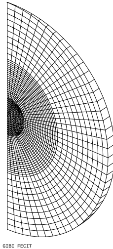
FIG. 6.1.1 – Maillage
