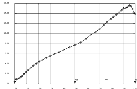
FIG. 2.3.11 – Ra = 10^6 , lignes de courant
