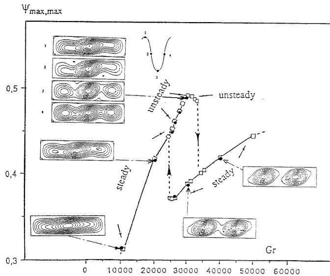
FIG. 2.5.2 – Diagramme de stabilité (d'après Le Garrec, S. & Magnaud, J-P. [2]).
