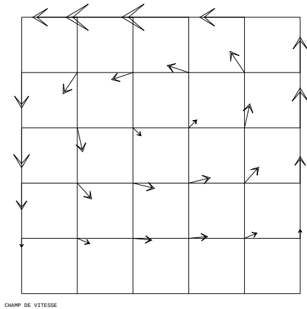
FIG. 7.2.1 – Champ de vitesse imposé sur maillage 5 \times 5
