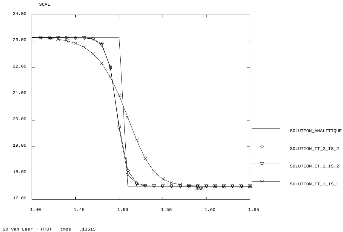
FIG. 5.1.13 – Enthalpie totale sur le choc.
