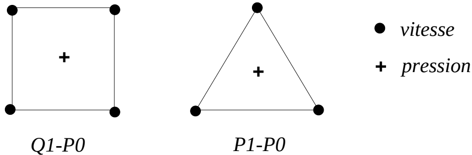
FIG. 2.4.1 – Eléments vitesse-pression Q1-P0 et P1-P0 de CASTEM2000
