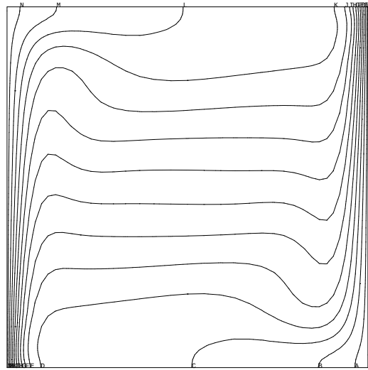
FIG. 2.3.3 – Ra = 10^6 , iso-températures
