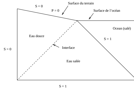
FIG. 6.3.1 – Salinité: schéma
