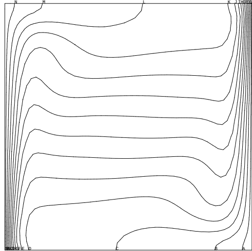
FIG. 2.3.9 – Ra = 10^6 , iso-températures
