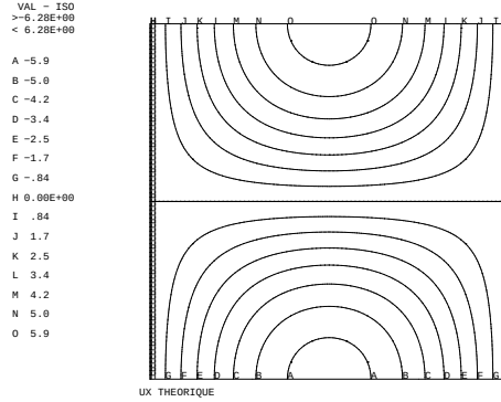
FIG. 2.4.3 – Composante u théorique
