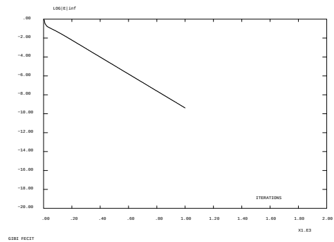
FIG. 2.4.10 – Historique de convergence pour atteindre l'état stationnaire
