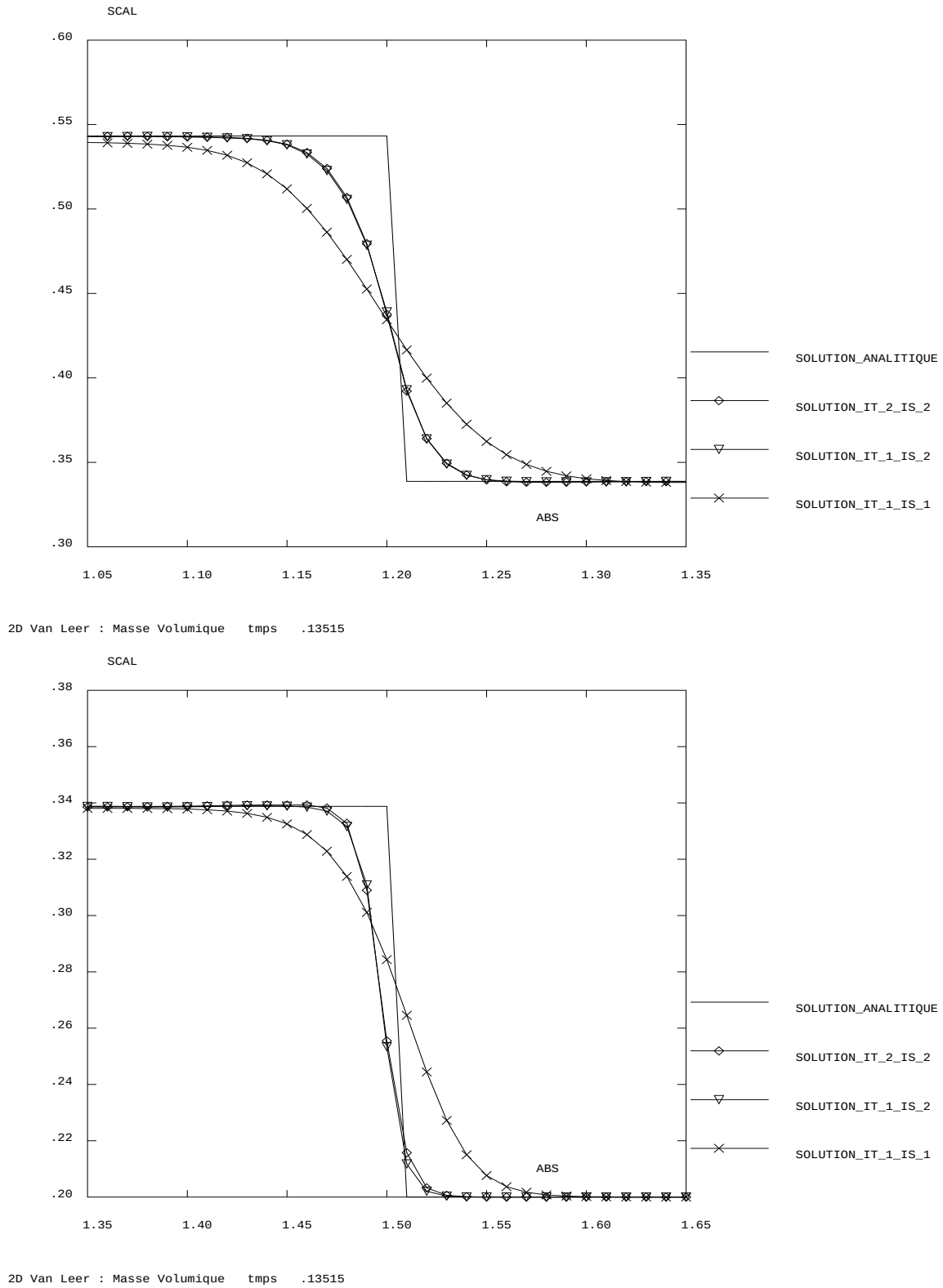
FIG. 5.1.5 – Masse volumique sur la surface de discontinuité et sur le choc.
