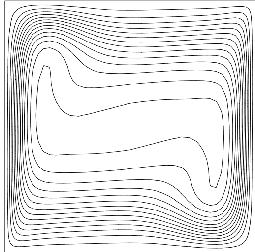
FIG. 2.3.3 – Ra = 10^6 , iso-températures
