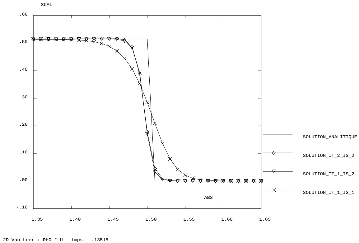
FIG. 5.1.10 – Débit au niveau du choc.
