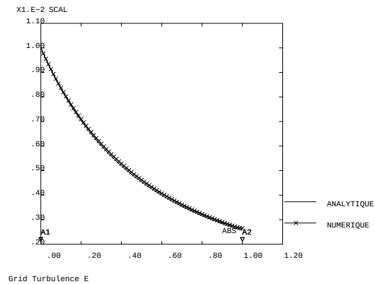
FIG. 3.1.4 – Comparaison sur \epsilon entre solutions numérique et analytique.
