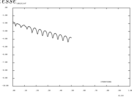
FIG. 2.3.12 – Ra = 10^6 , histoire de convergence
