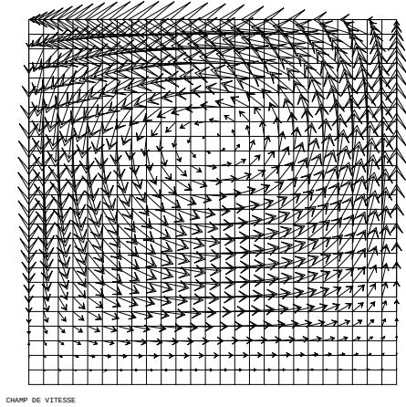
FIG. 7.2.3 – Champ de vitesse imposé sur maillage 25 \times 25
