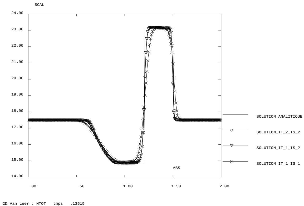
FIG. 5.1.11 – Enthalpie totale.
