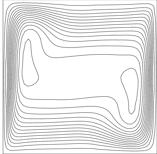
FIG. 2.3.9 – Ra = 10^6 , iso-températures
