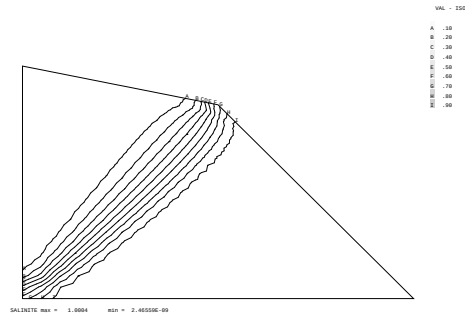
FIG. 6.3.2 – Salinité: Champ de salinité
