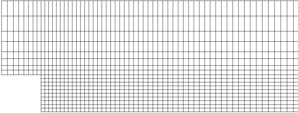
FIG. 2.2.3 – détail du maillage constitué de 2928 éléments et 3123 nœuds
