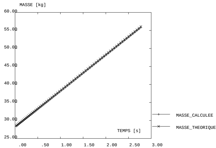
FIG. 5.3.2 – Evolution de la masse dans l'enceinte : prédiction numérique et théorie
