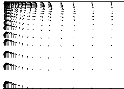
FIG. 3.3.5 – Détail du champ de vitesse (coin supérieur gauche)
