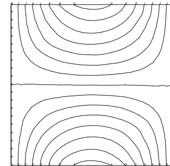
FIG. 2.4.16 – Champ de vitesse (composante u ) calculé
