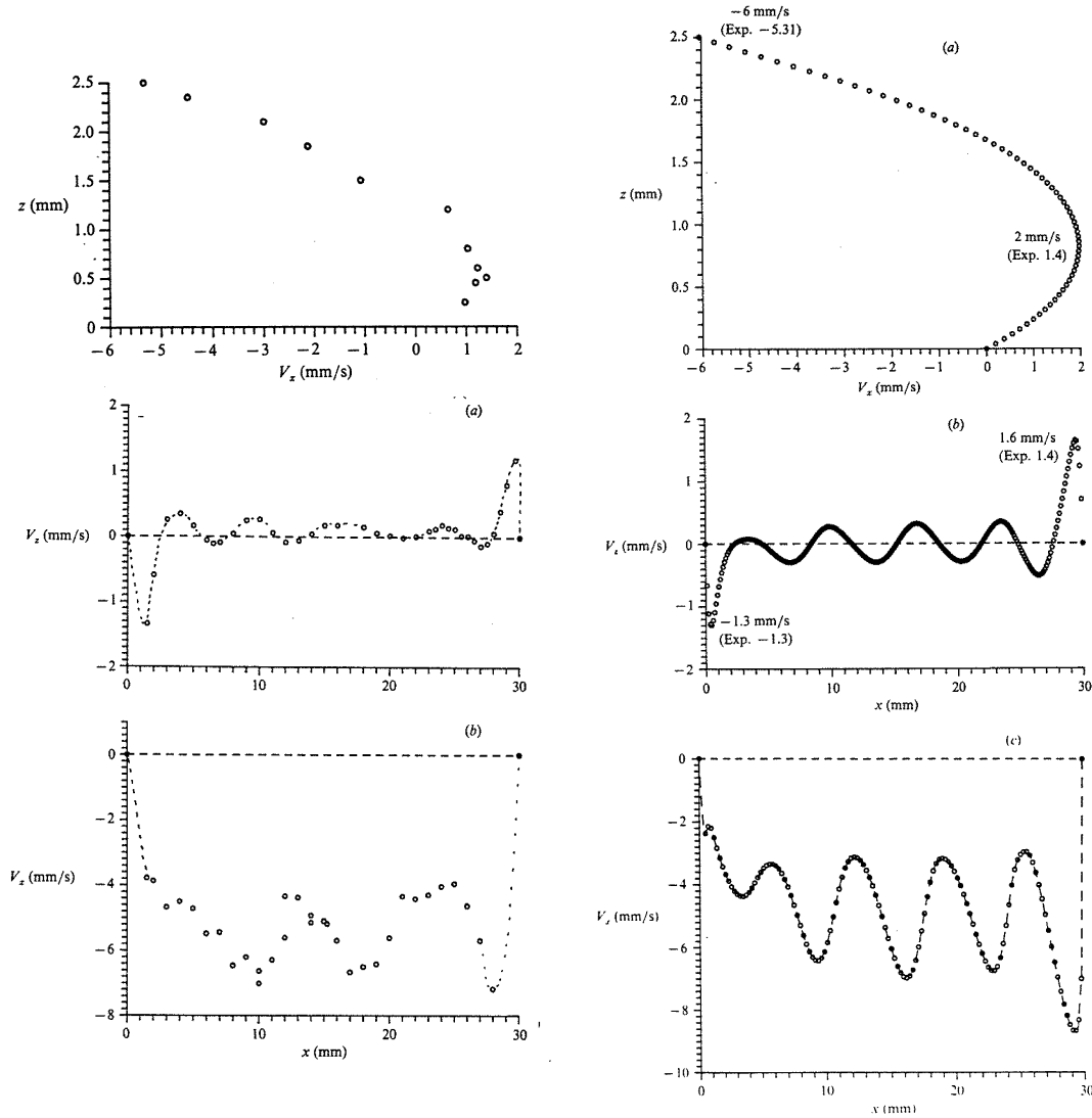
FIG. 2.6.5 – (a) Profil de vitesse horizontale u_x(z) sur la médiane verticale de la cavité, (b) composante verticale de la vitesse u_z(x) sur une ligne horizontale à z = 1.35 mm, et (c) composante horizontale de la vitesse u_x(x) sur la surface. A droite, la simulation numérique de l'écoulement avec Pr=4.24 , Ra=8600 , Ma=15200 et A=12 ; ces conditions correspondent à l'expérience, à gauche (d'après Villers, D. & Platten, J.K. [1]).
