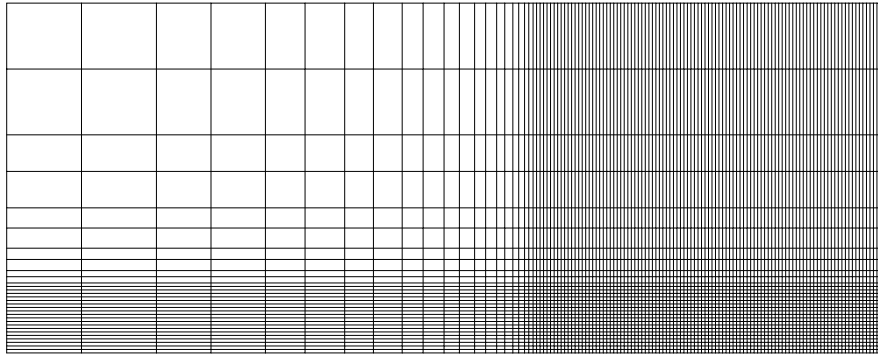
FIG. 2.1.3 – Maillage constitué de 3600 éléments et 3751 nœuds
