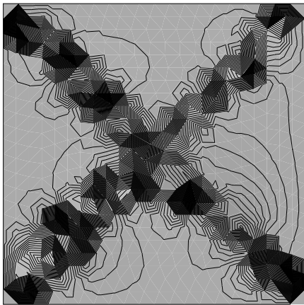
FIG. 1.6.5 – Erreur \epsilon = (T_{num} - T_{ex})/T_{ex} sur triangles : \text{Max } |\epsilon| = 4. \times 10^{-4}
