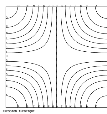
FIG. 2.4.2 – Pression théorique
