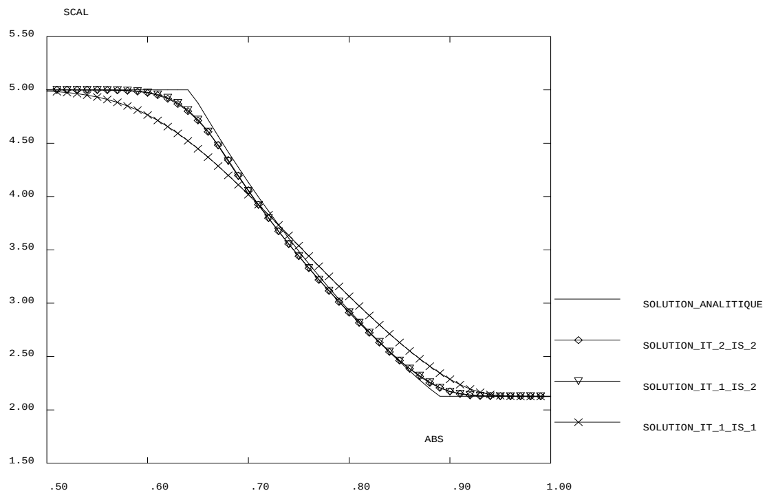
FIG. 5.1.6 – Pression le long du tube et dans la zone de détente.
