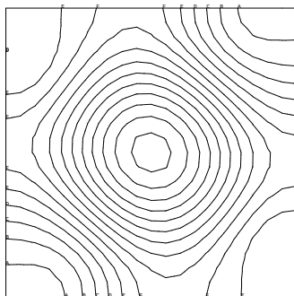
FIG. 2.4.11 – Champ de pression calculé
