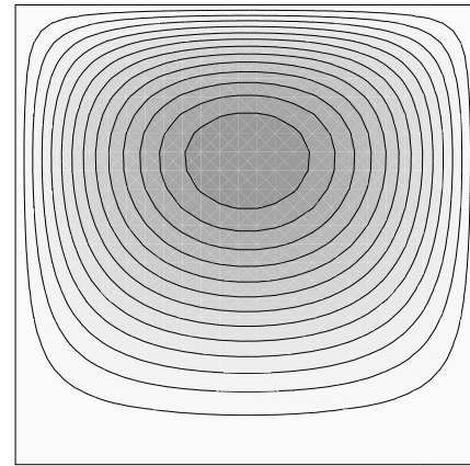
FIG. 7.2.2 – Fonction de courant calculée sur maillage 5 \times 5
